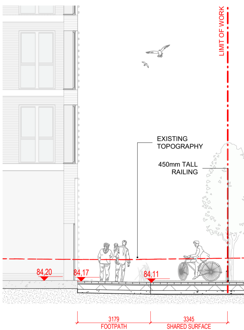
7 A-Section 07 1: 100 @A1
